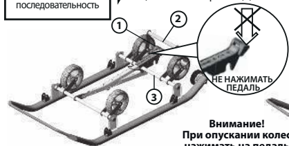
Рис. 3 Механизм выдвигающих колес
