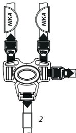
Рис. 2 Крепление ремней безопасности
