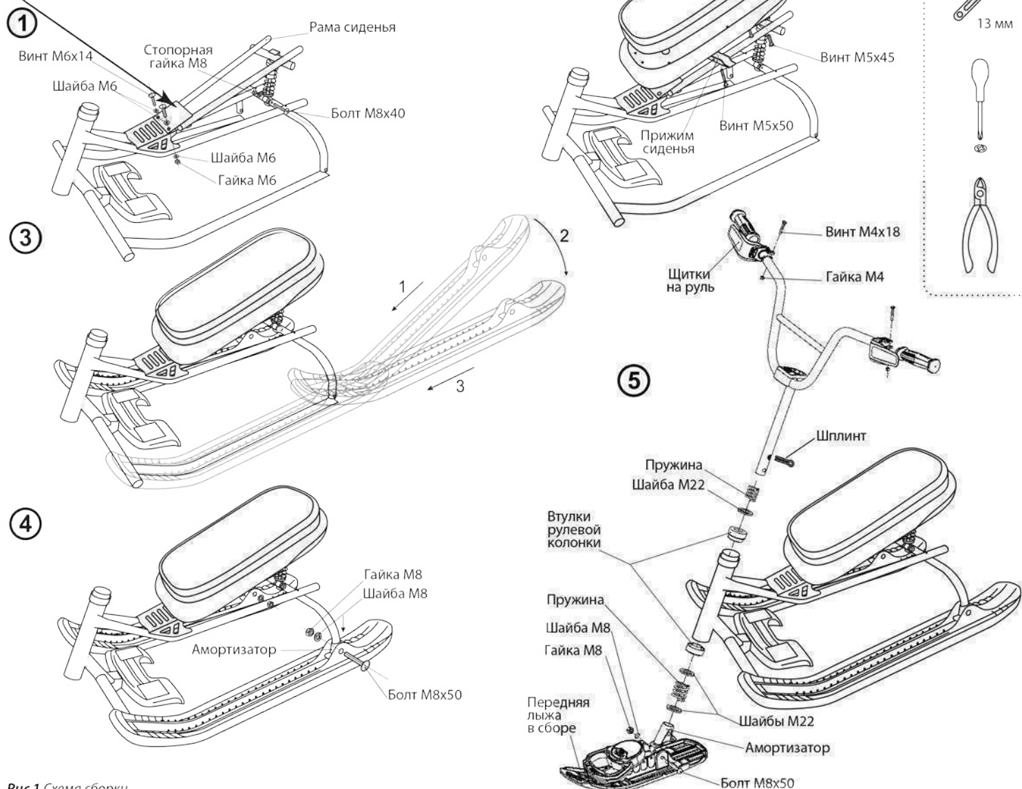
Рис 1 Схема сборки
