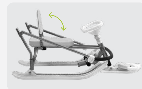
Складная ручка-толкатель
