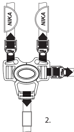
Рис. 2 Крепление ремней безопасности.
