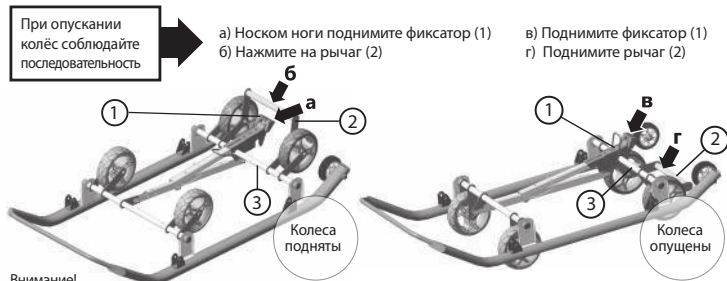
Рис. 3 Механизм выдвижных колёс
