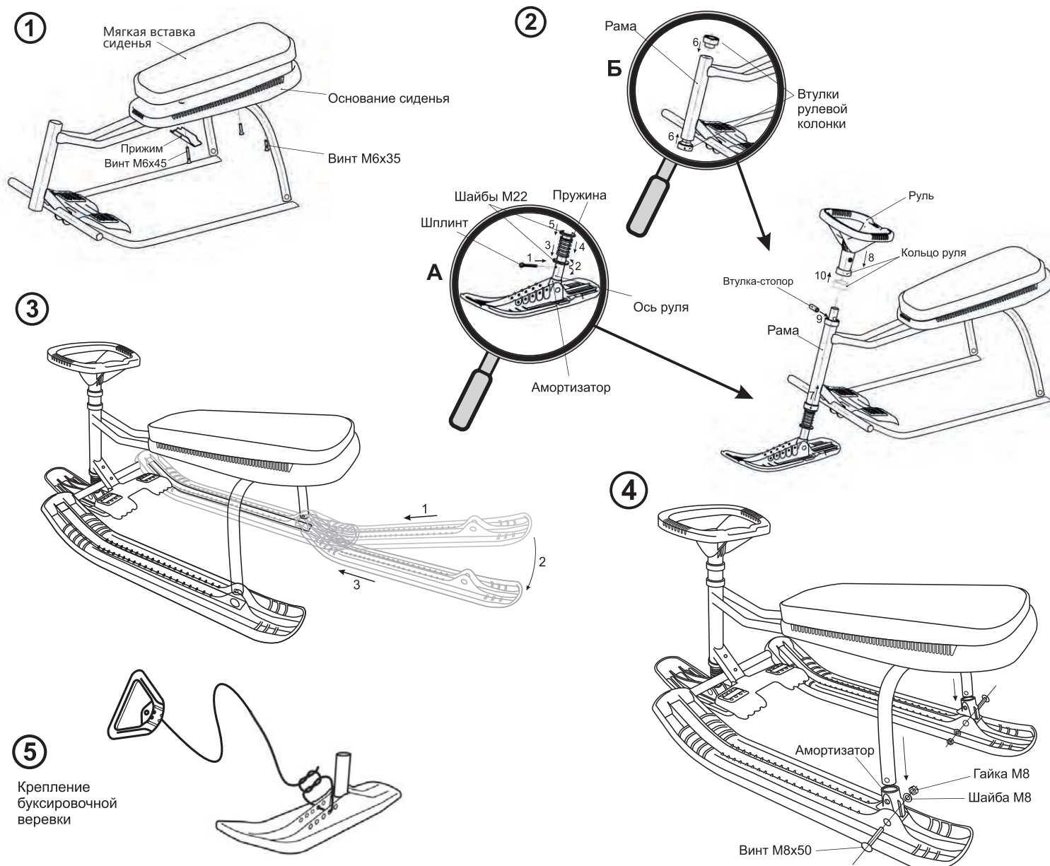
Рис. 1 Схема сборки
