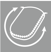
круговая молния
