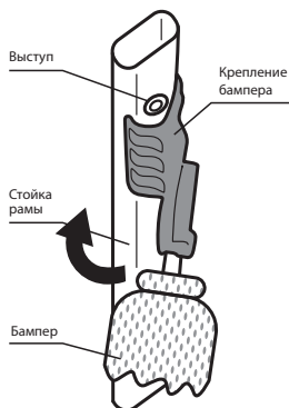
Рис. 4 Крепление бампера
