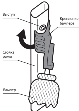
Рис. 4 Крепление бампера
