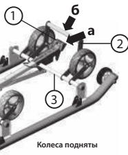
Рис. 3 Механизм выдвижных колес
