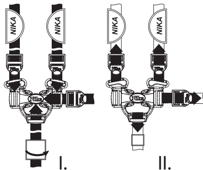
Рис. 2 Крепление ремней безопасности
