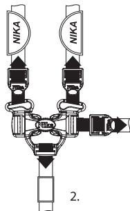
рис. 2 Крепление ремней безопасности.
